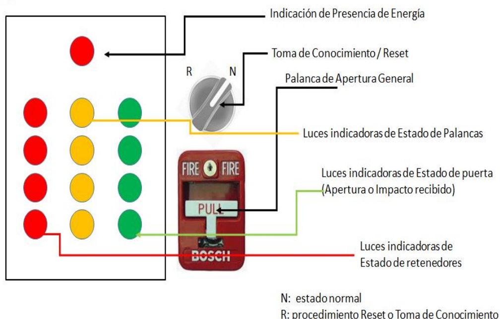
PANEL DE CONTROL RELOJ CONTROL
